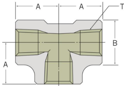
Tee
